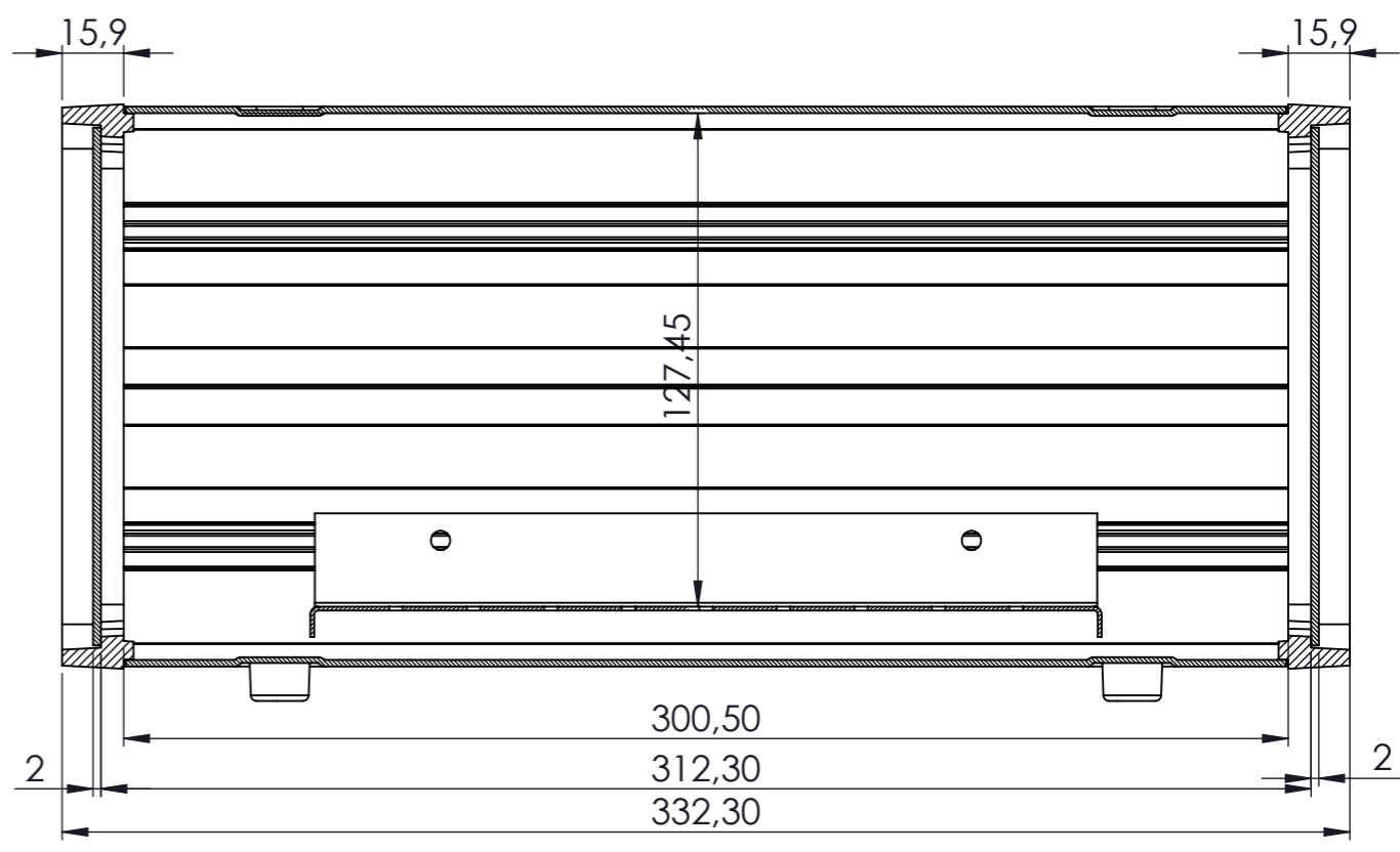
KESIT A-A
