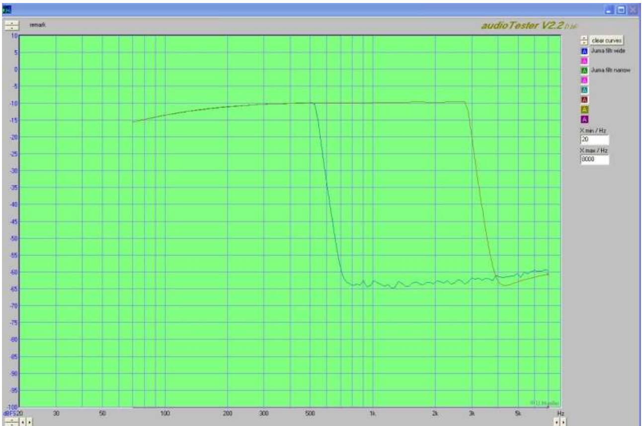
Wykres działania LPF - MAX7400
