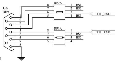
X1M尾部DB9口
