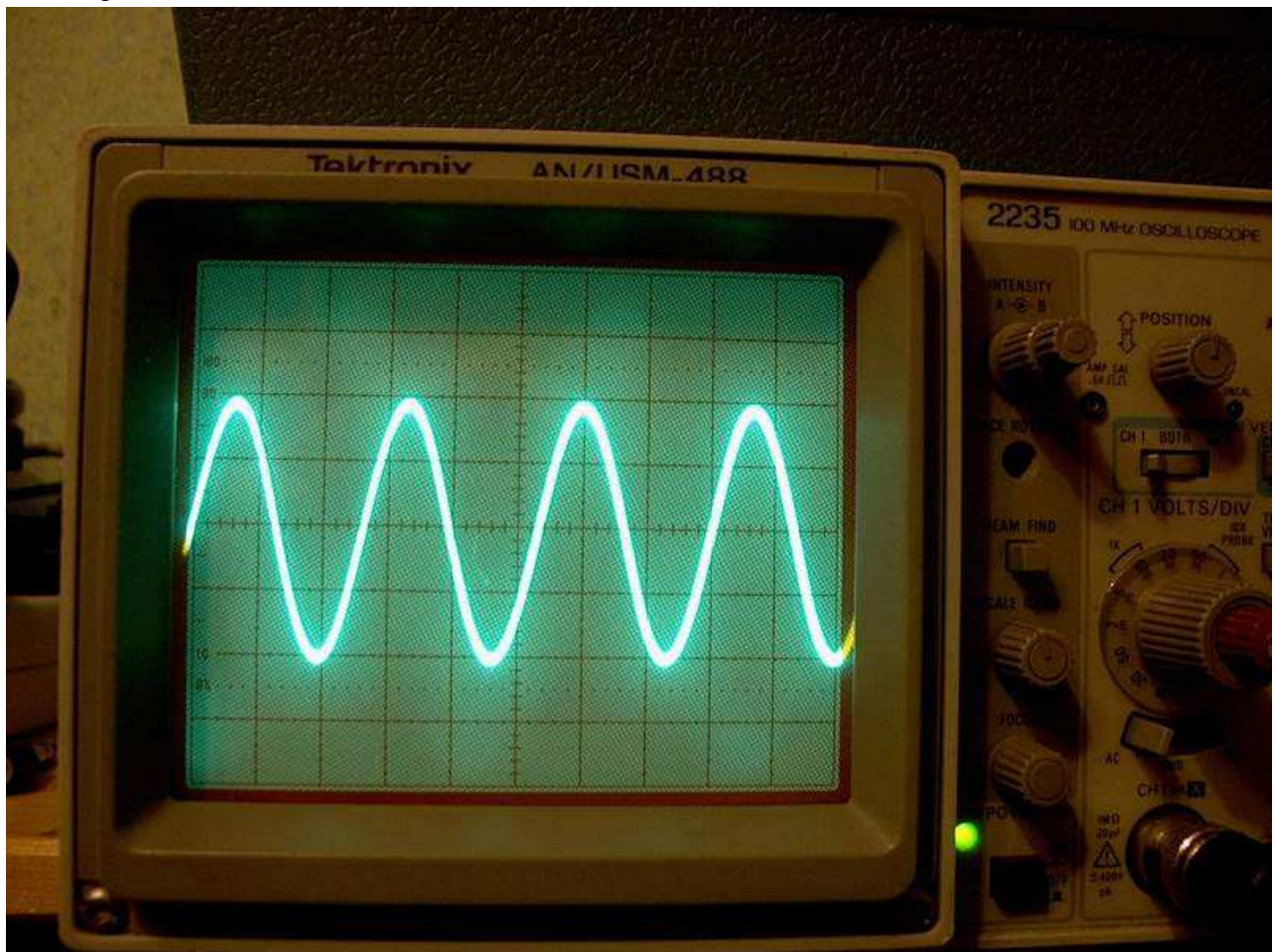
sygnał wejściowy IF,RX (-20dBm) 3,5Mhz sygnał po dedektorze wejścia polifazera 1,2,3,4 400mV p-p , sygnał VFO 3,5Mhz x 4 poziom -10dBm
