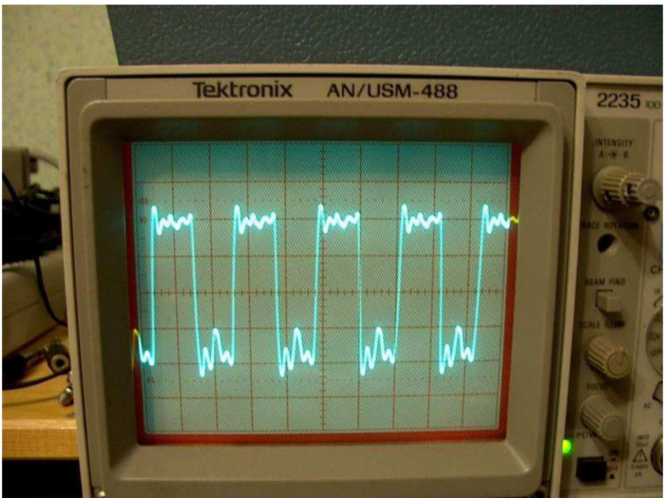
Przebieg n.11 układ U2-74AC164 , VFO 35Mhz - 10dBm
