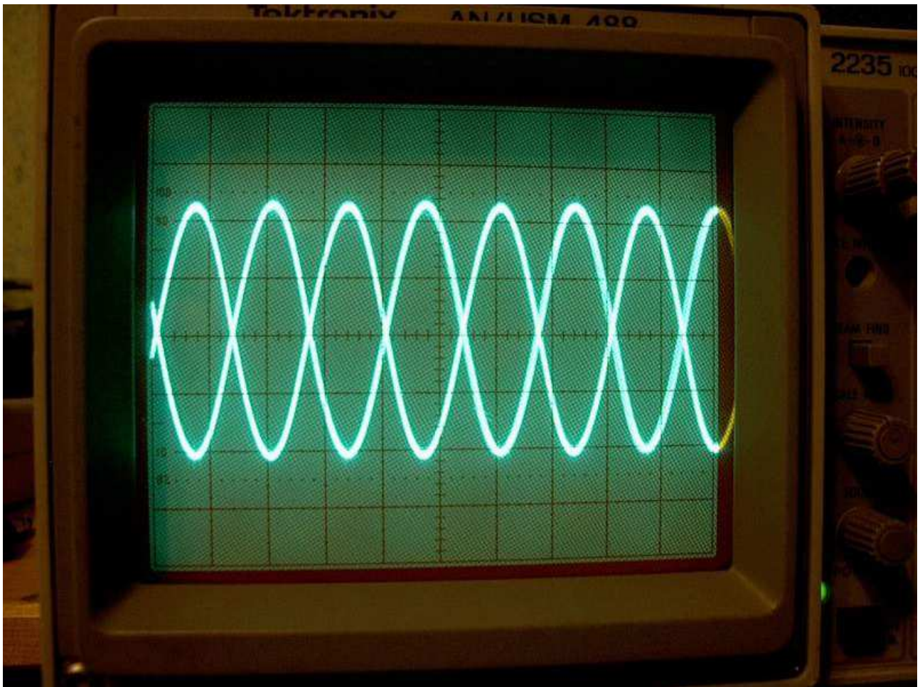
wyjście z polifazera n.5,6 - 1 kanał n. 7,8 - 2 kanał oscyloskopu
