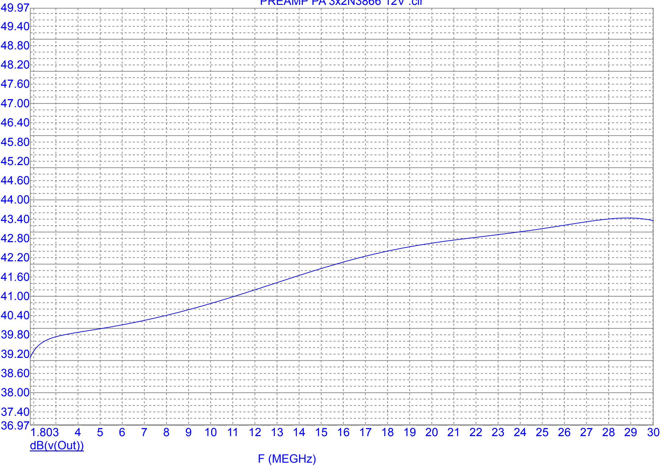
PREAMP PA 3x2N3866 12V .cir
